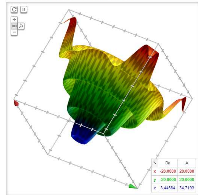
Grafico per \sqrt{x^2+y^2}+3\cos(\sqrt{x^2+y^2})+5
