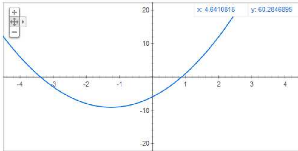
Grafico per 2x^2+5x-6
